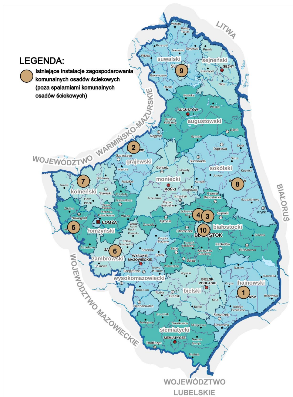
Rysunek 3.41. Rozmieszczenie instalacji zagospodarowania komunalnych osadów ściekowych (poza spalarniami komunalnych osadów ściekowych) w 2019 r.; numeracja zgodna z tab. 3.37.
